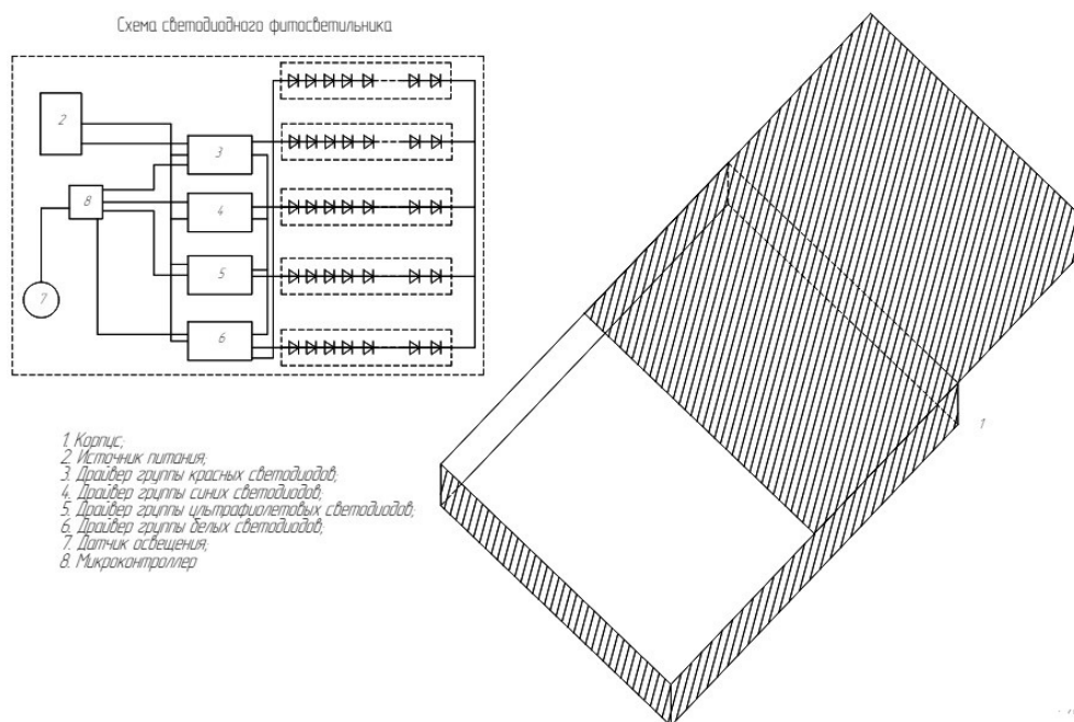
Рис. 1 Схема светодиодного фитосветильника
