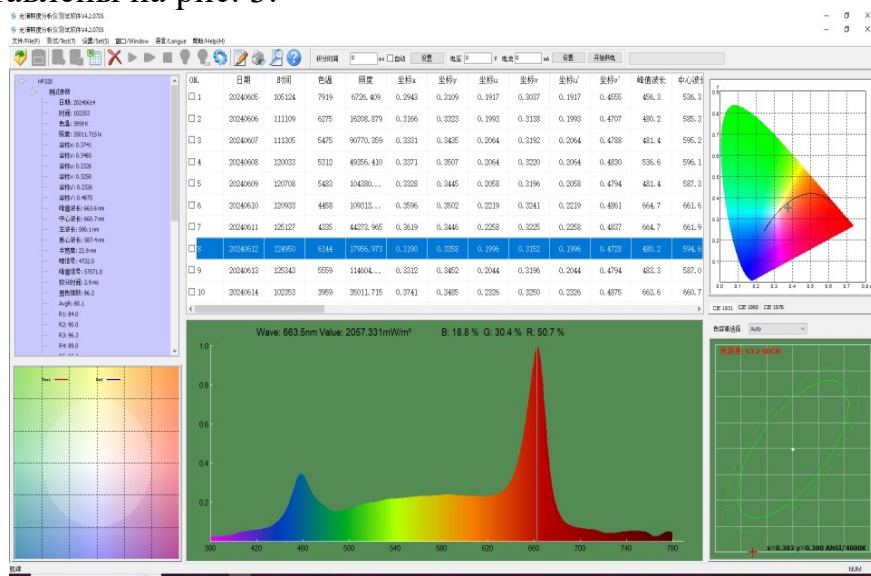
Рис. 3 Исследование спектрального состава в течении суток
